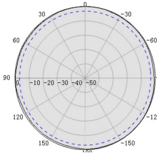
Horizontal Beamwidth
